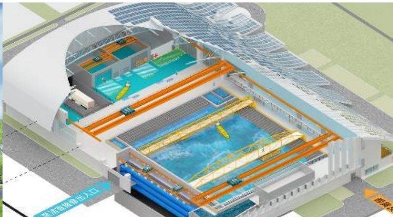
等角透視圖
